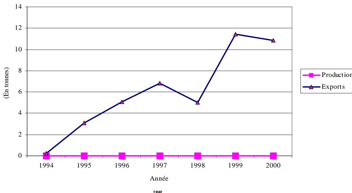
Figure 1 Ouganda : production et exportation d'or, 1994-2000
